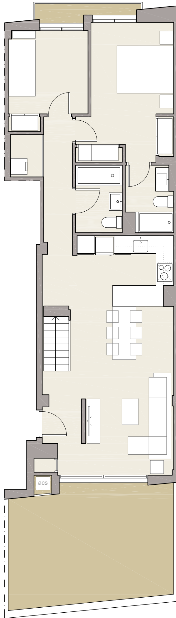
PLANTA VIVIENDA
